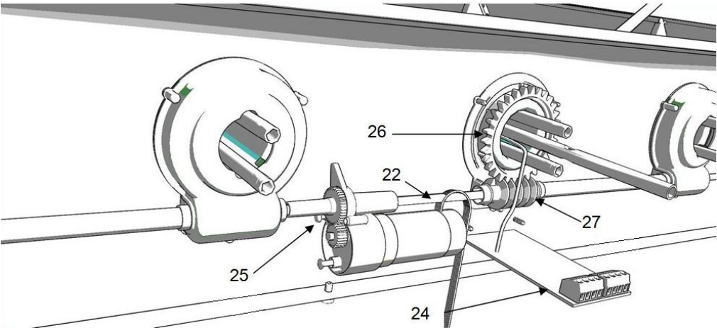
Fig. 7 - Particolare catena cinematica
