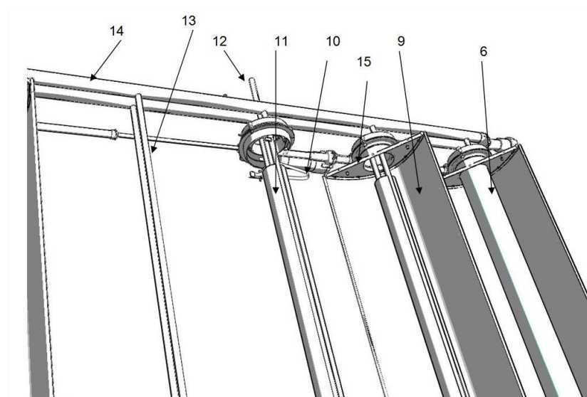
Fig. 2 - Particolare specchi concentratori
