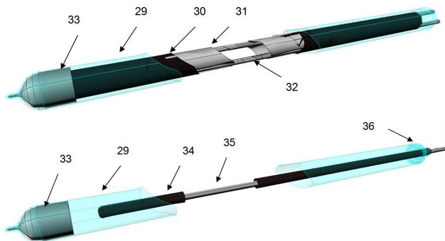
Fig. 10 - Struttura di due differenti tipologie di tubi assorbitori dewar. Quello superiore integralmente in vetro e quello inferiore con un passante vetro metallo.
