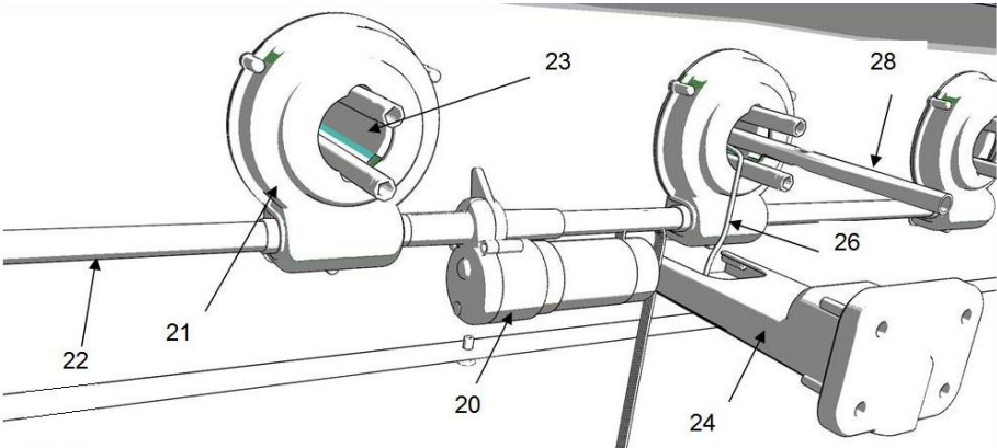
Fig. 7 - Particolare catena cinematica
