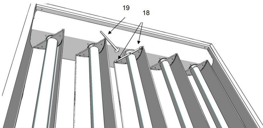
Fig. 6 - Movimento specchi
