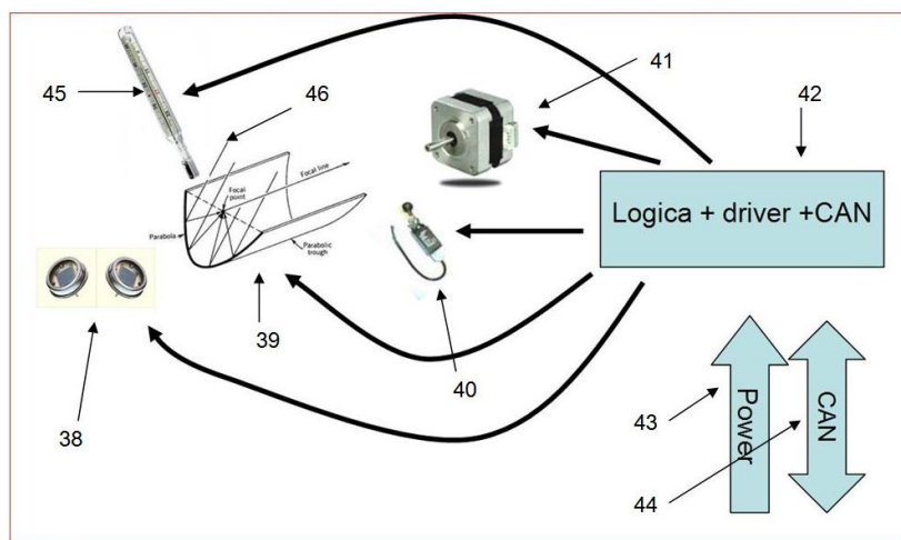
Fig. 11 – Interazione componenti nel caso singolo pannello
