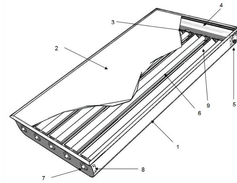
Fig. 1- Disegno CAD SOL INVICTUS
