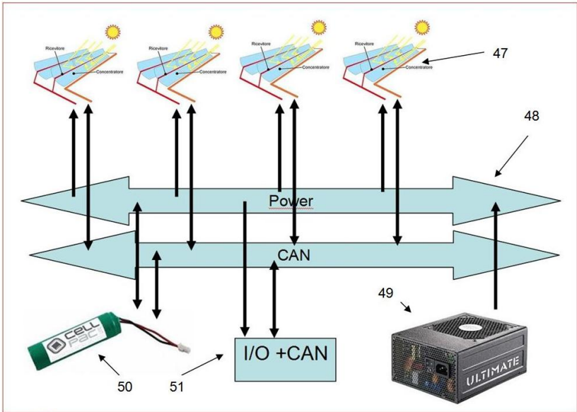
Fig. 12 - Interazione componenti nel caso rete di pannelli
