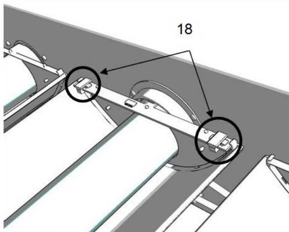
Fig. 5 - Presenza due detector sullo specchio centrale
